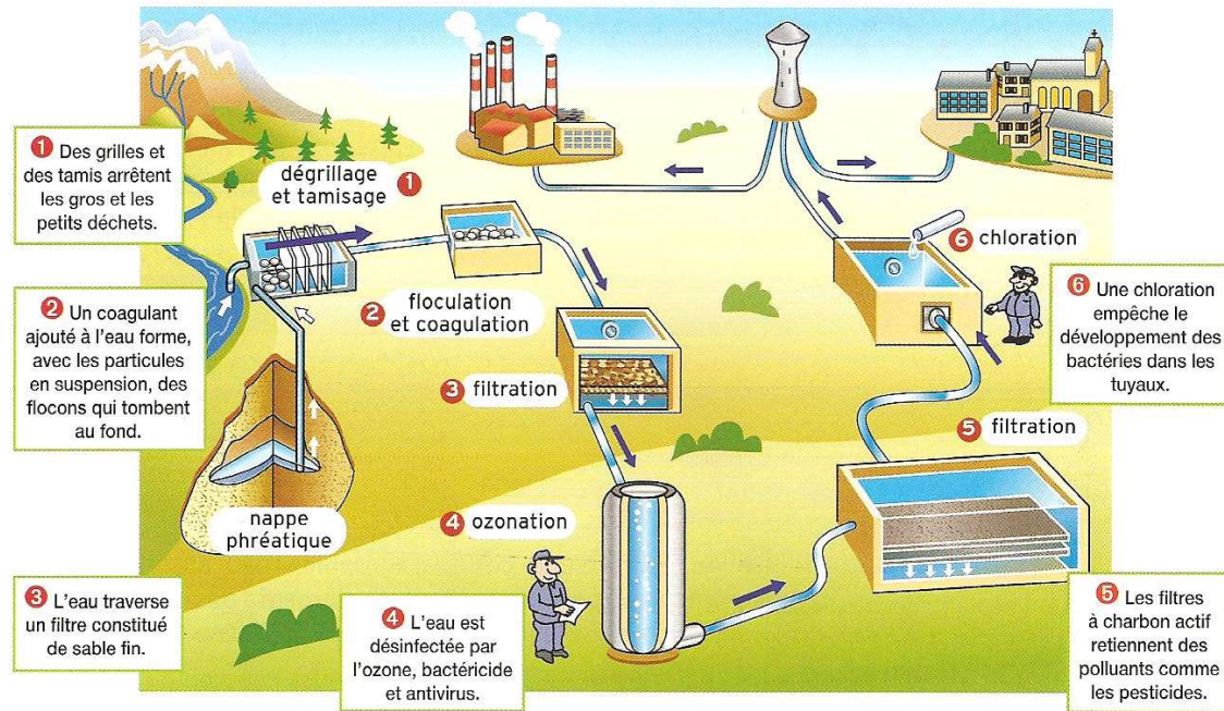
Principe de fonctionnement d'une station de traitement
